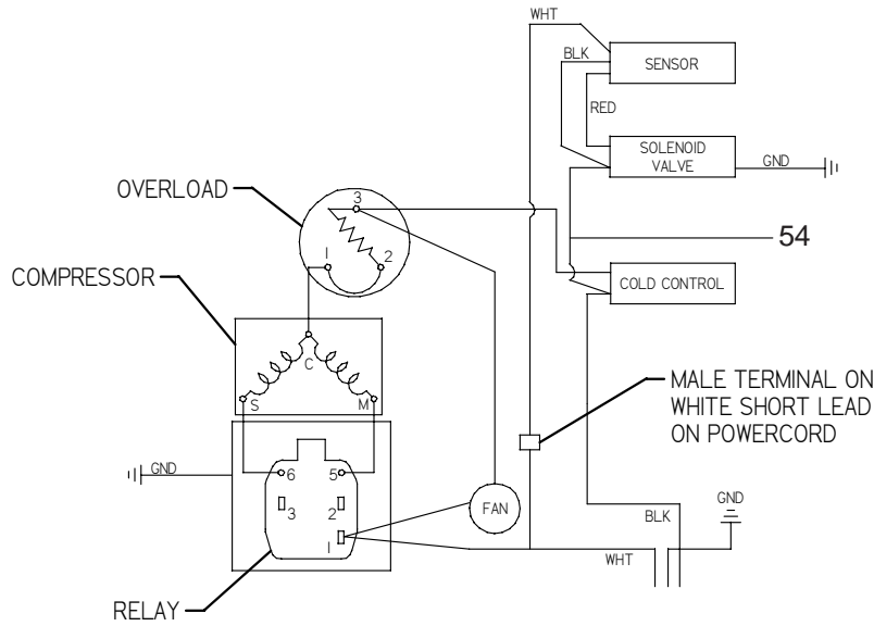
WIRING DIAGRAM - HTV8EE 115V El ESQUEMA que ALAMBRA - HTV8EE 115V DIAGRAMME qui TELEGRAPHIE - HTV8EE 115V
