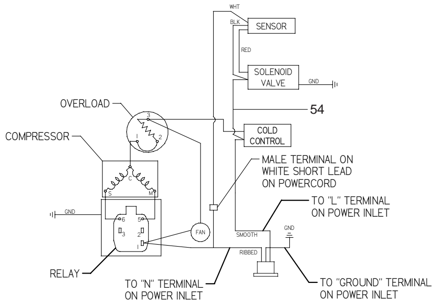
WIRING DIAGRAM - HTV8EE 220V El ESQUEMA que ALAMBRA - HTV8EE 220V DIAGRAMME qui TELEGRAPHIE - HTV8EE 220V
